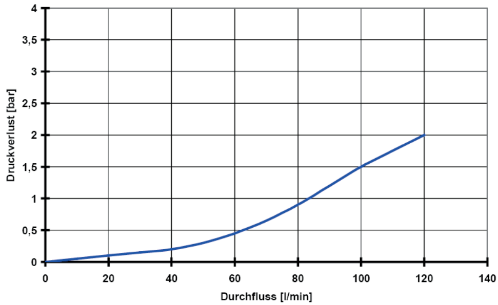
RVM/UM, Druckverlust für Wasser bei 20 °C
