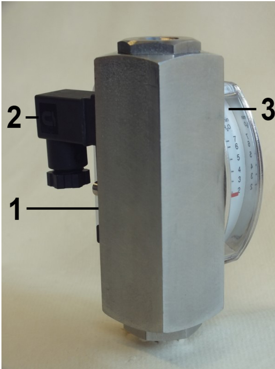
Abb. 1: Strömungswächter RVM/UA-L2
