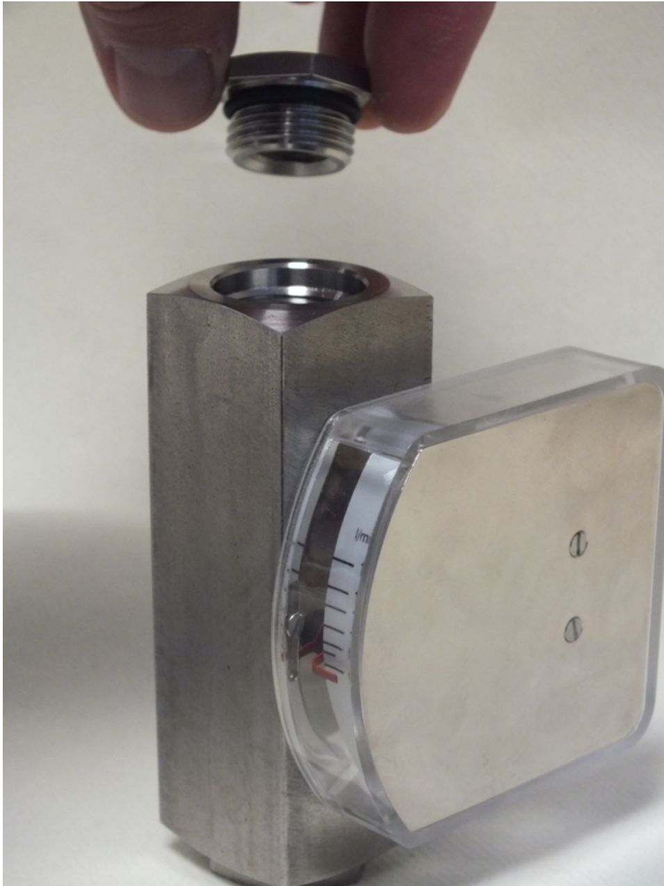
Abb. 58: Verschraubung (Ausgang) einsetzen
