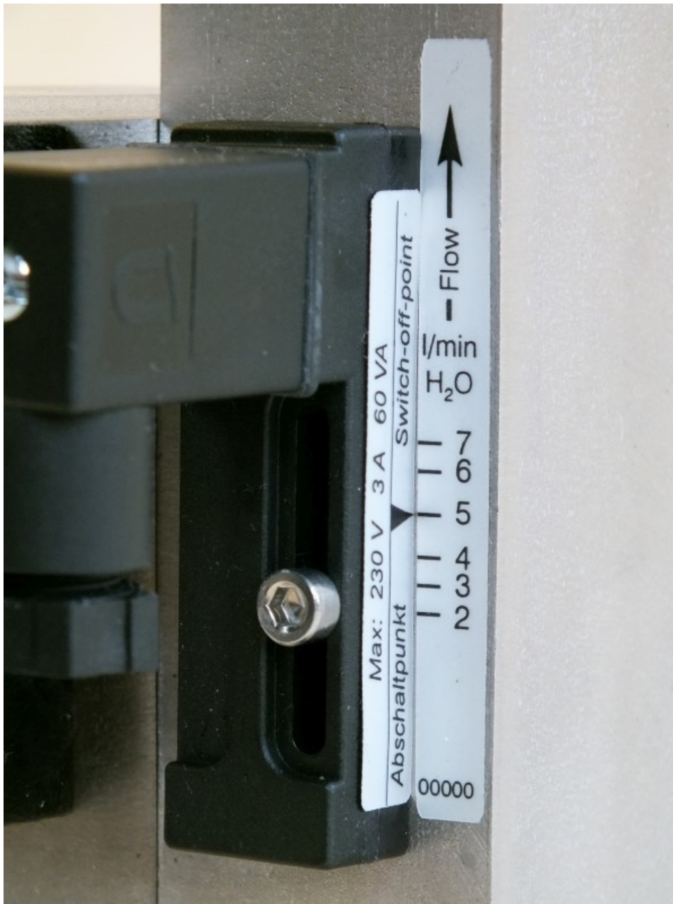
Abb. 4: Körperskala
