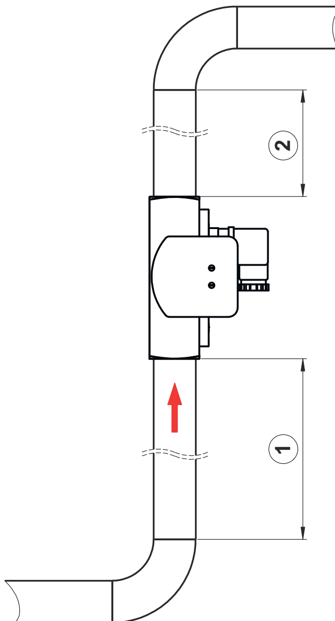
Abb. 7: Beruhigungsstrecken
