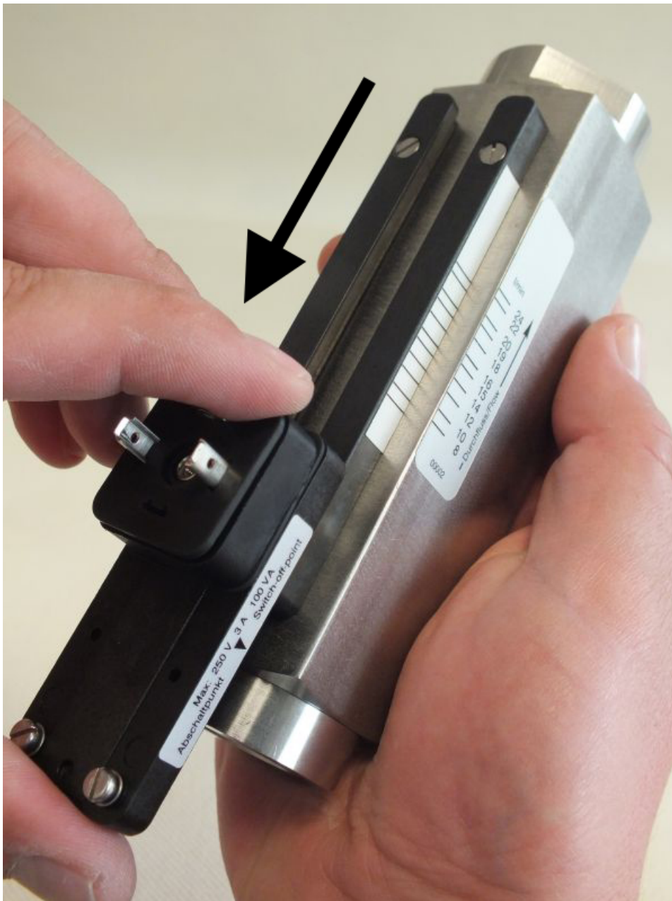
Abb. 67: Schaltkontakt aus Führung schieben
