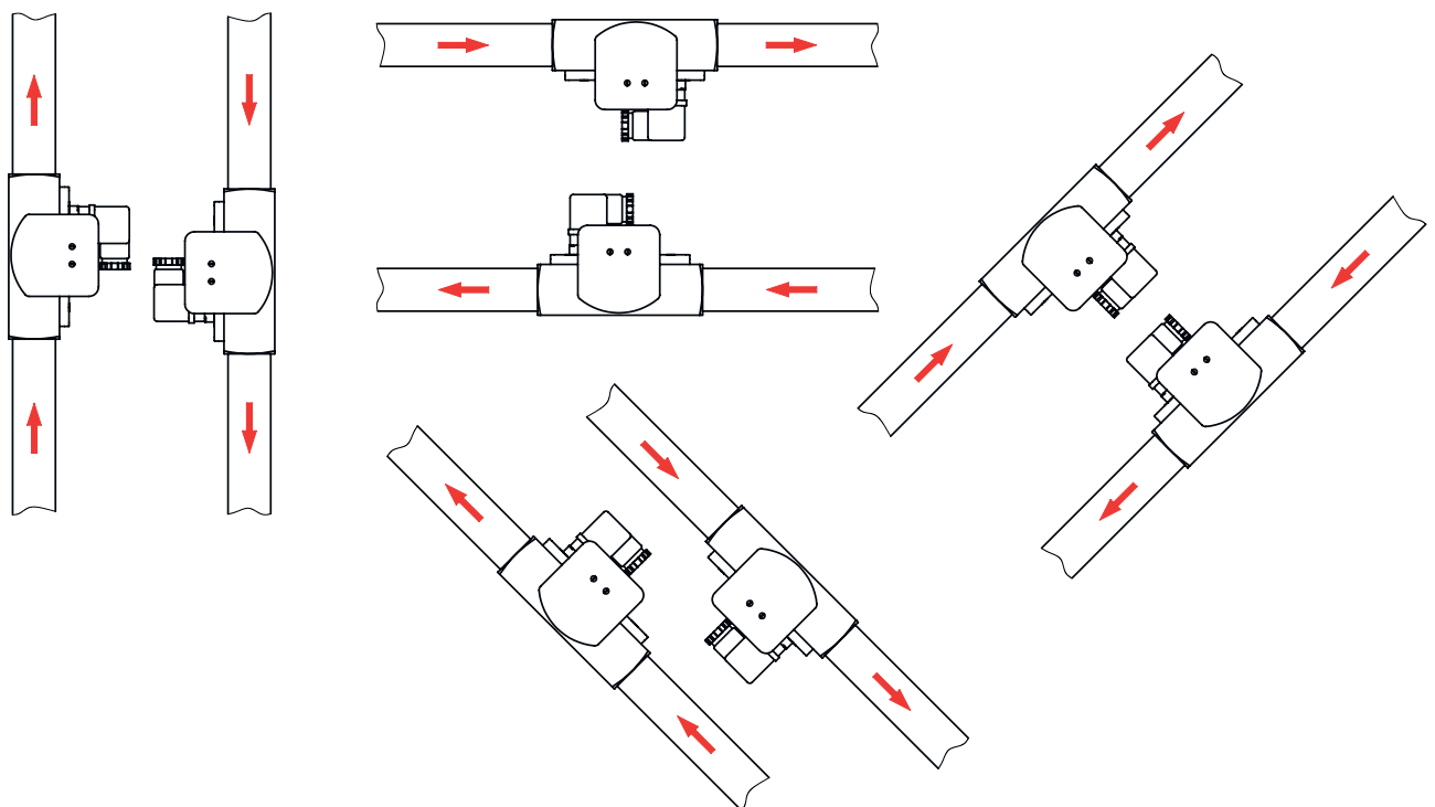
Abb. 6: Einbauposition/Durchflussrichtung
