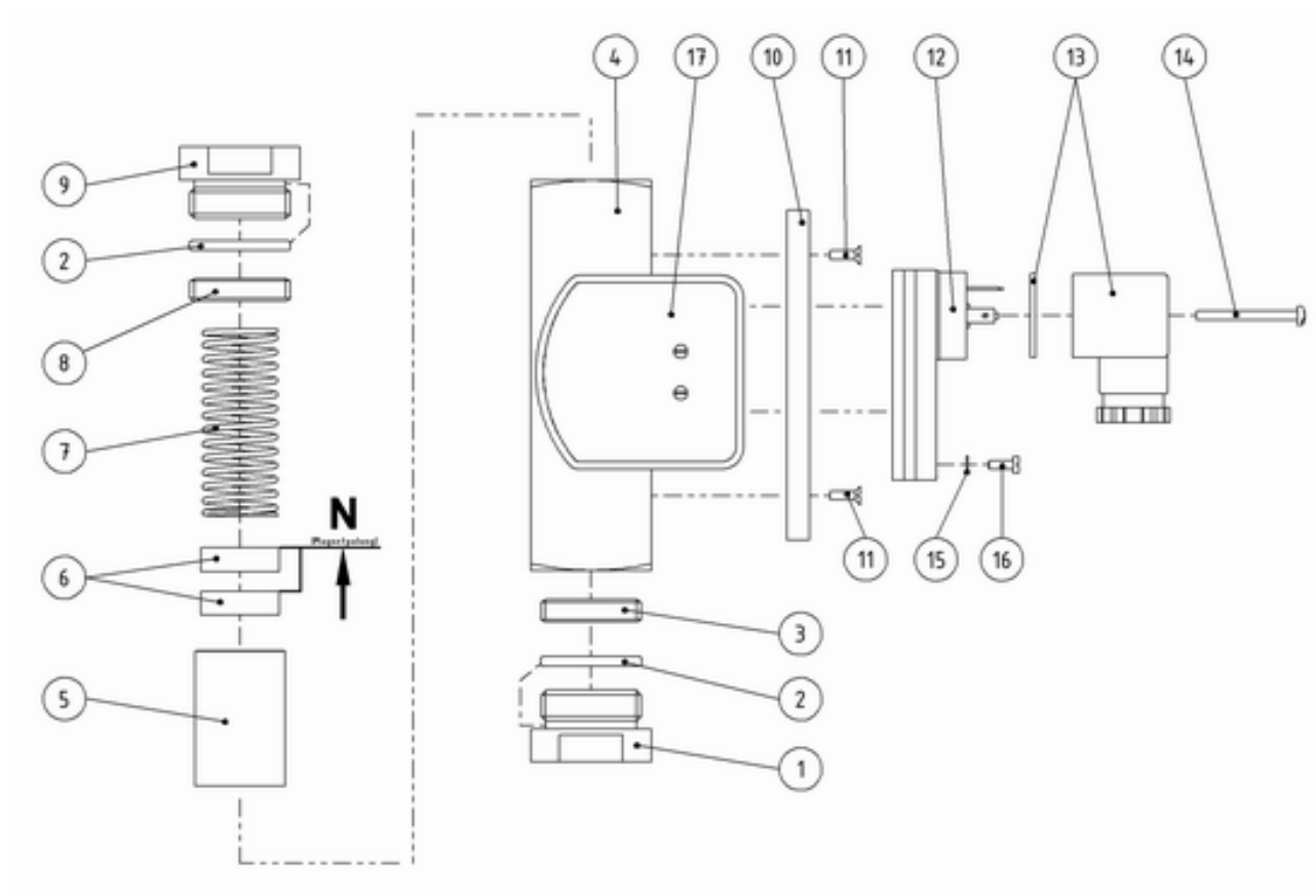
Abb. 74: Ersatzteilzeichnung RVM/UA-L1 Basics
