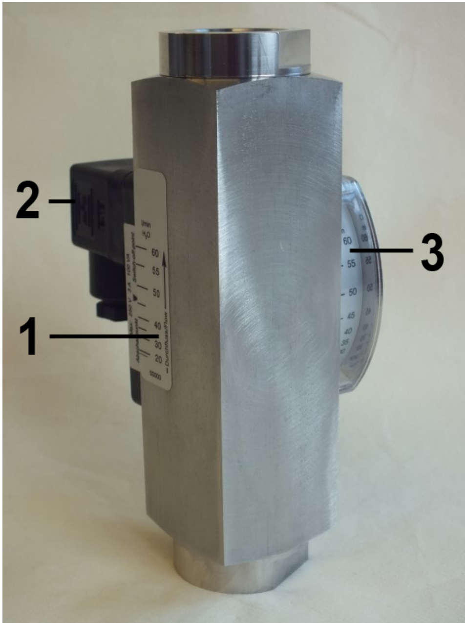
Abb. 1: Strömungswächter RVM/UA-L1
