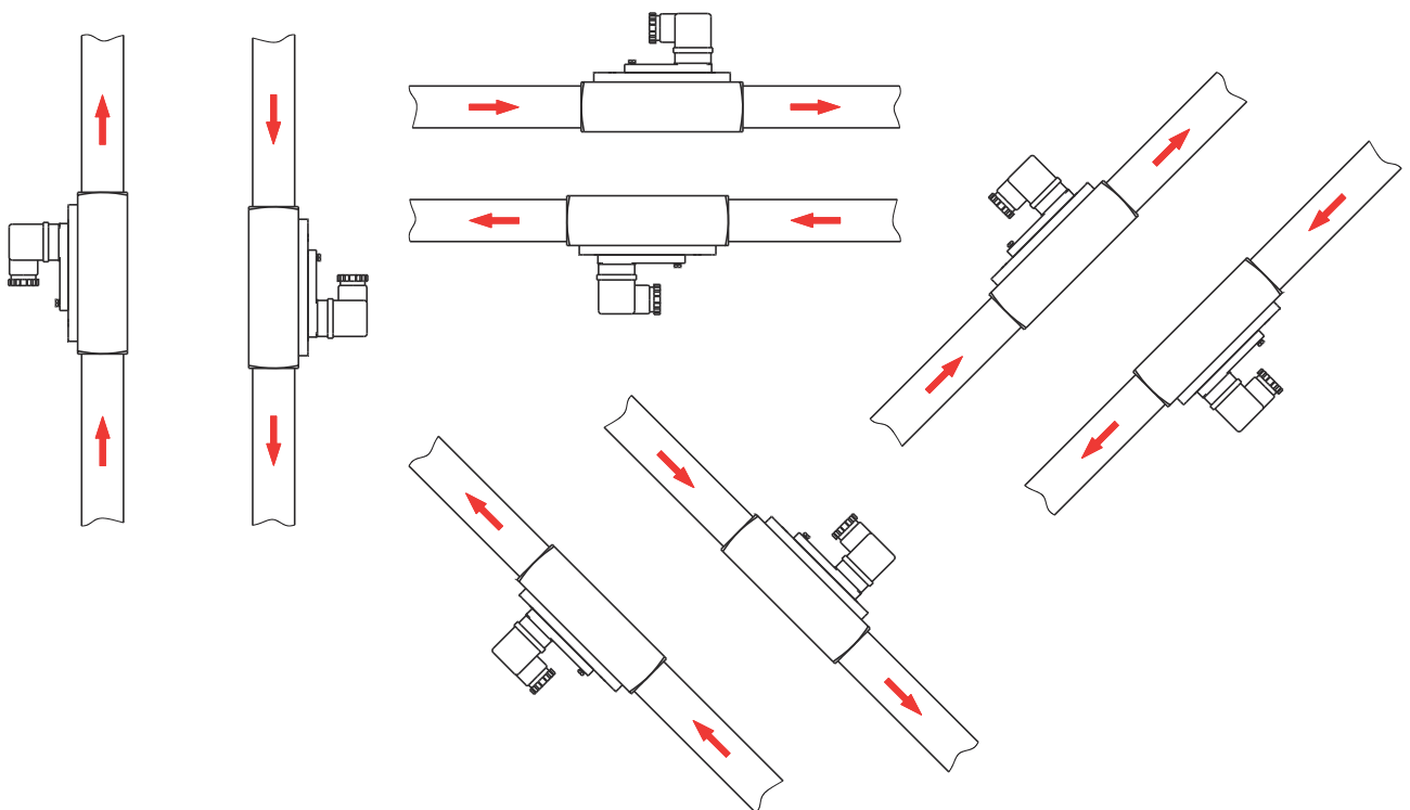
Abb. 5: Einbauposition/Durchflussrichtung
