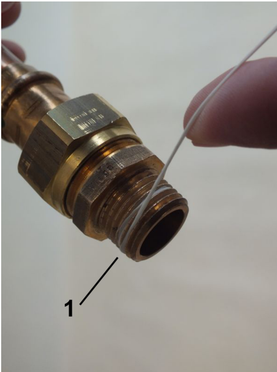
Abb. 8: Dichtfaden aufbringen
