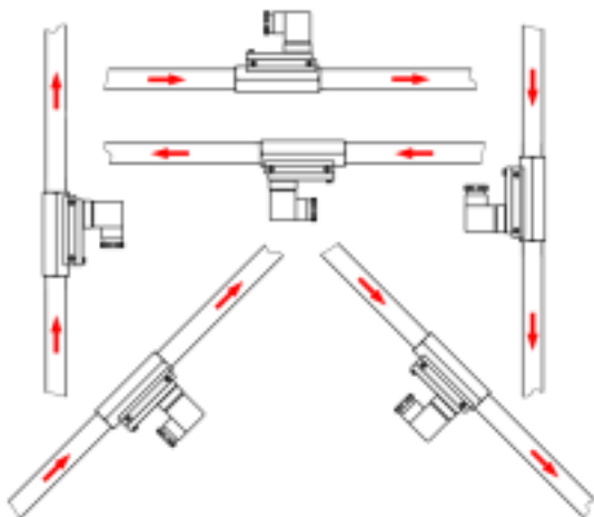
Abb. 5: Einbauposition/Durchflussrichtung
