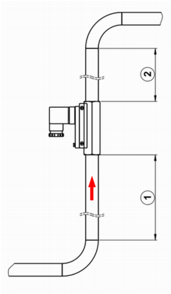
Abb. 6: Beruhigungsstrecken
