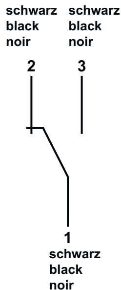
Abb. 21: Zustand des Kontaktes bei Gerät ohne Durchfluss
