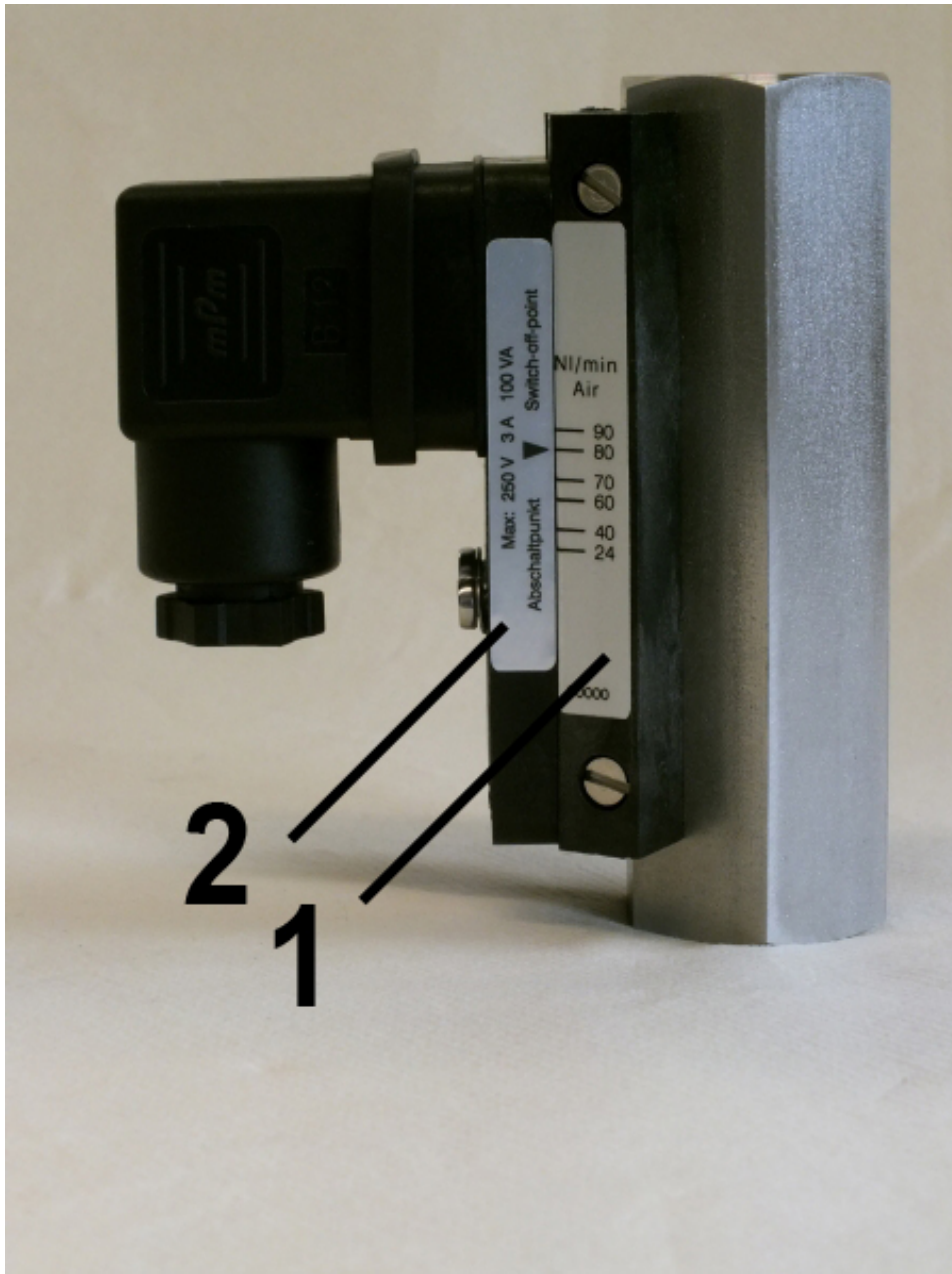
Abb. 1: Strömungswächter RVM/U-L2 30x70
