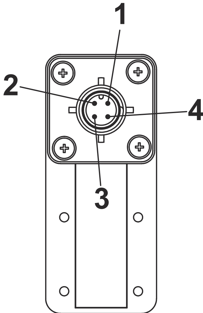
Abb. 16: Pin-Belegung Gerätestecker M12x1
