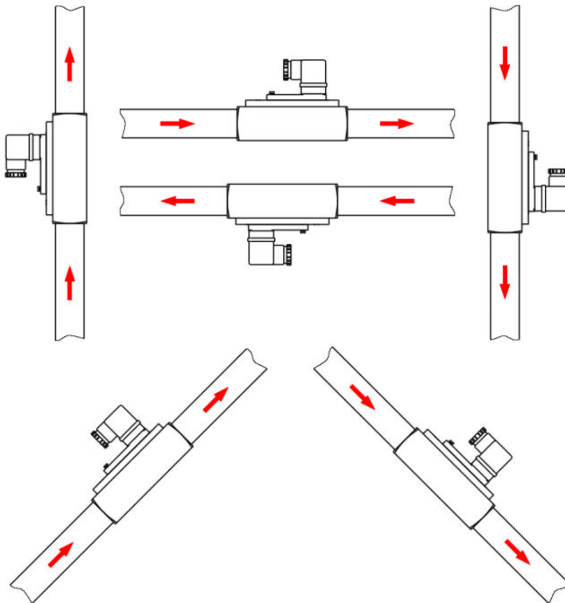
Abb. 5: Einbauposition/Durchflussrichtung
