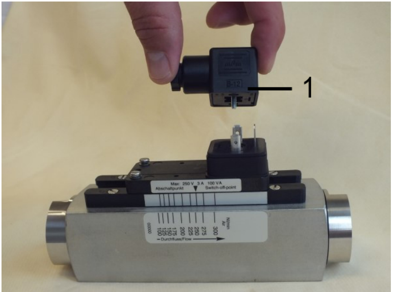
Abb. 66: Steckerdose abziehen
