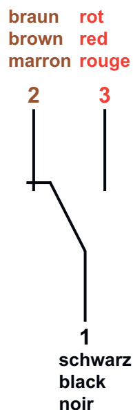
Abb. 24: Zustand des Kontaktes bei Gerät ohne Durchfluss
