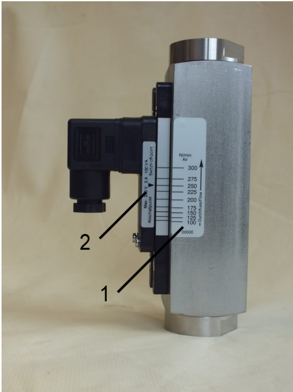
Abb. 1: Strömungswächter RVM/U-L1
