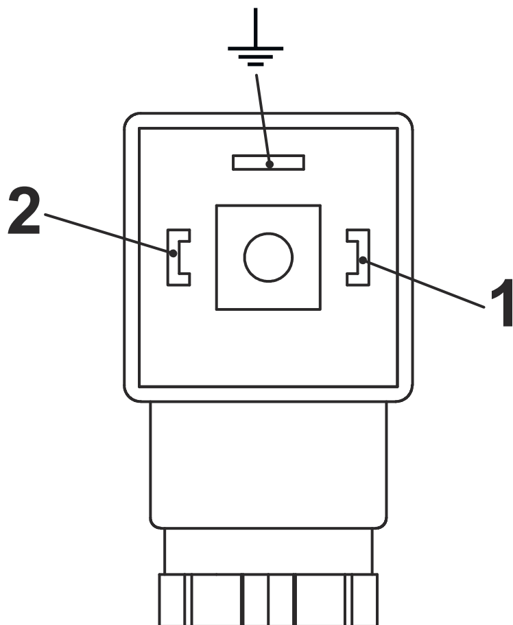
Abb. 13: Pin-Belegung Steckerdose Schließer (Erde-Anschluss nicht genutzt)
