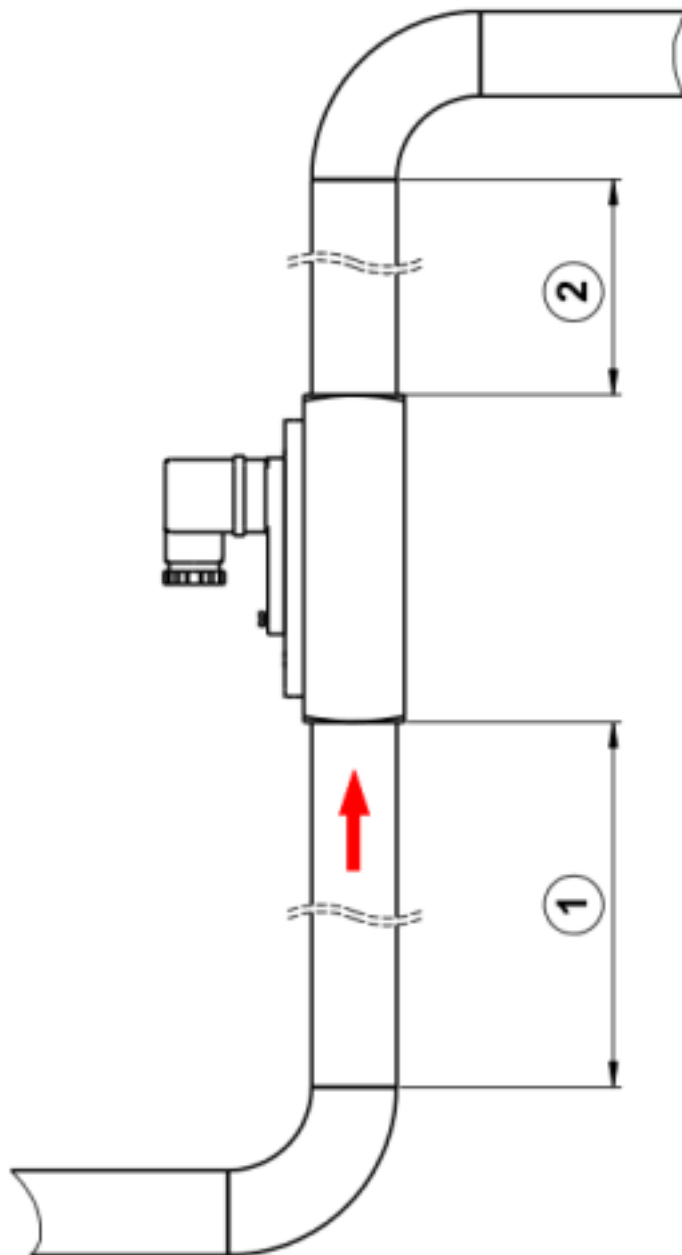
Abb. 6: Beruhigungsstrecken
