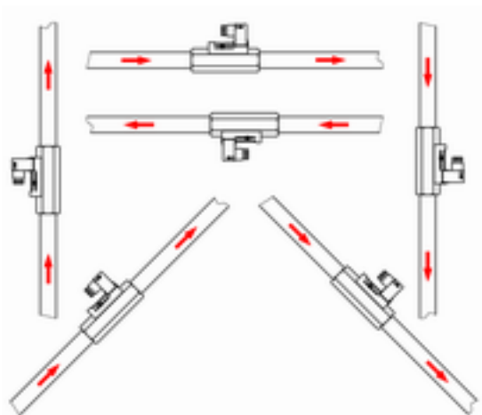
Abb. 5: Einbauposition/Durchflussrichtung
