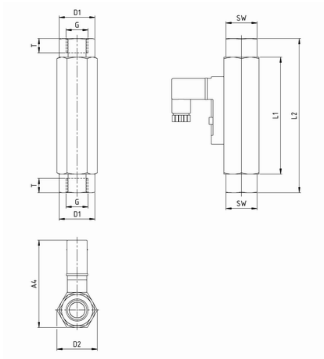
Abb. 62: RVM/U-2 mit Schaltkontakt 15x50
