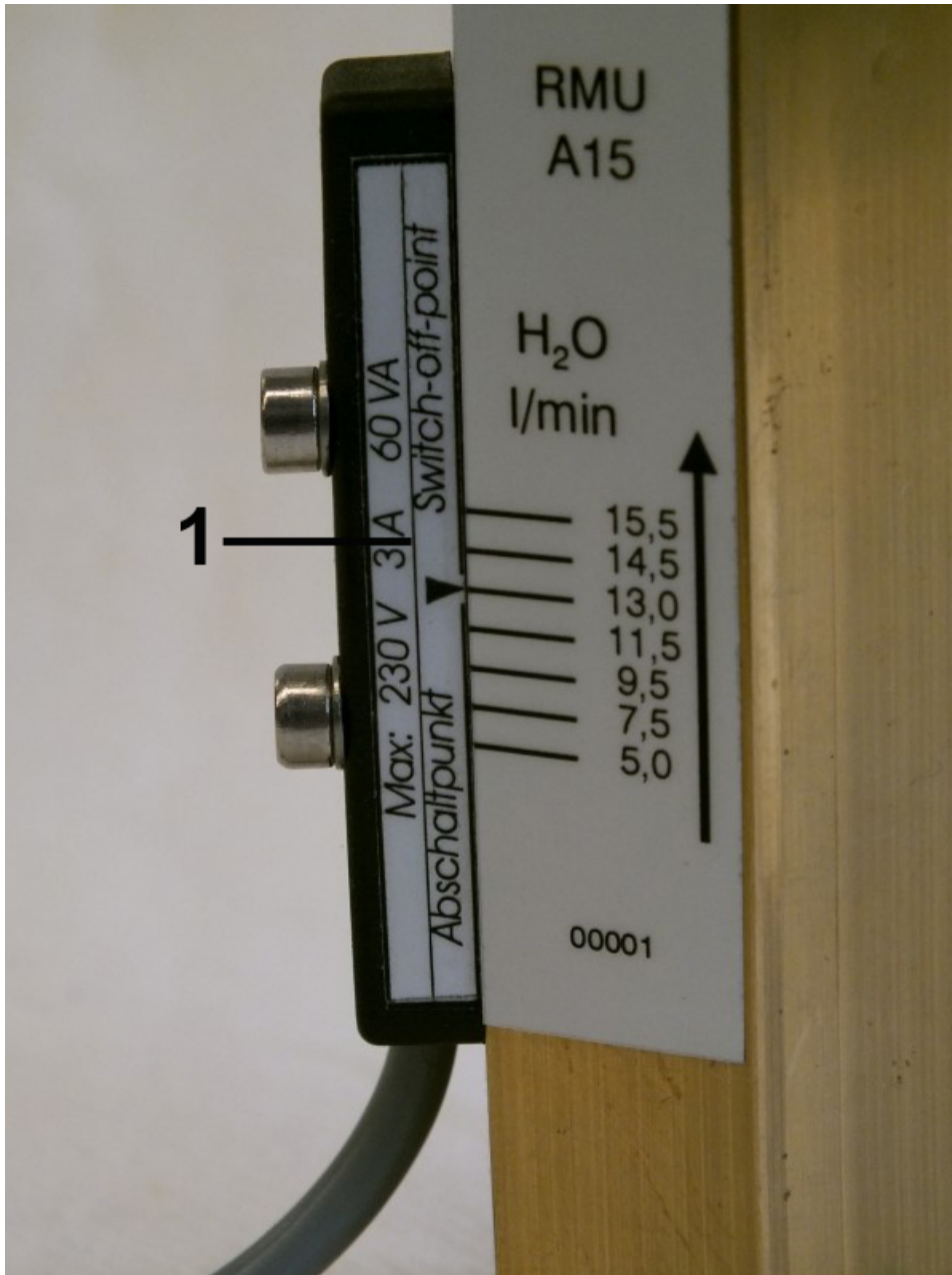
Abb. 3: Schaltkontakt mit Anschlusskabel
