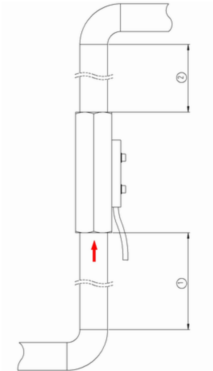
Abb. 6: Beruhigungsstrecken
