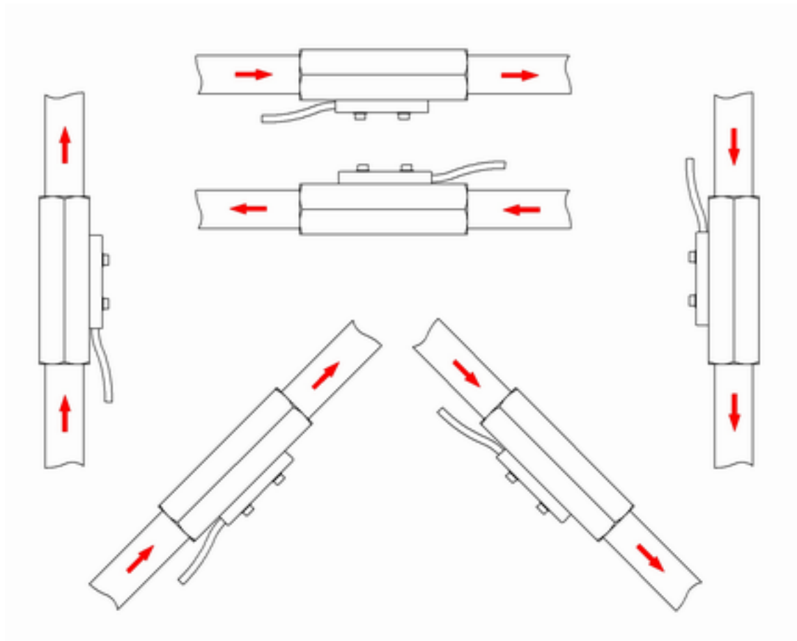
Abb. 5: Einbauposition/Durchflussrichtung
