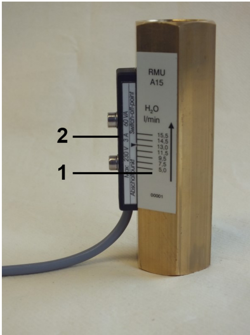
Abb. 1: Strömungswächter RMU-A
