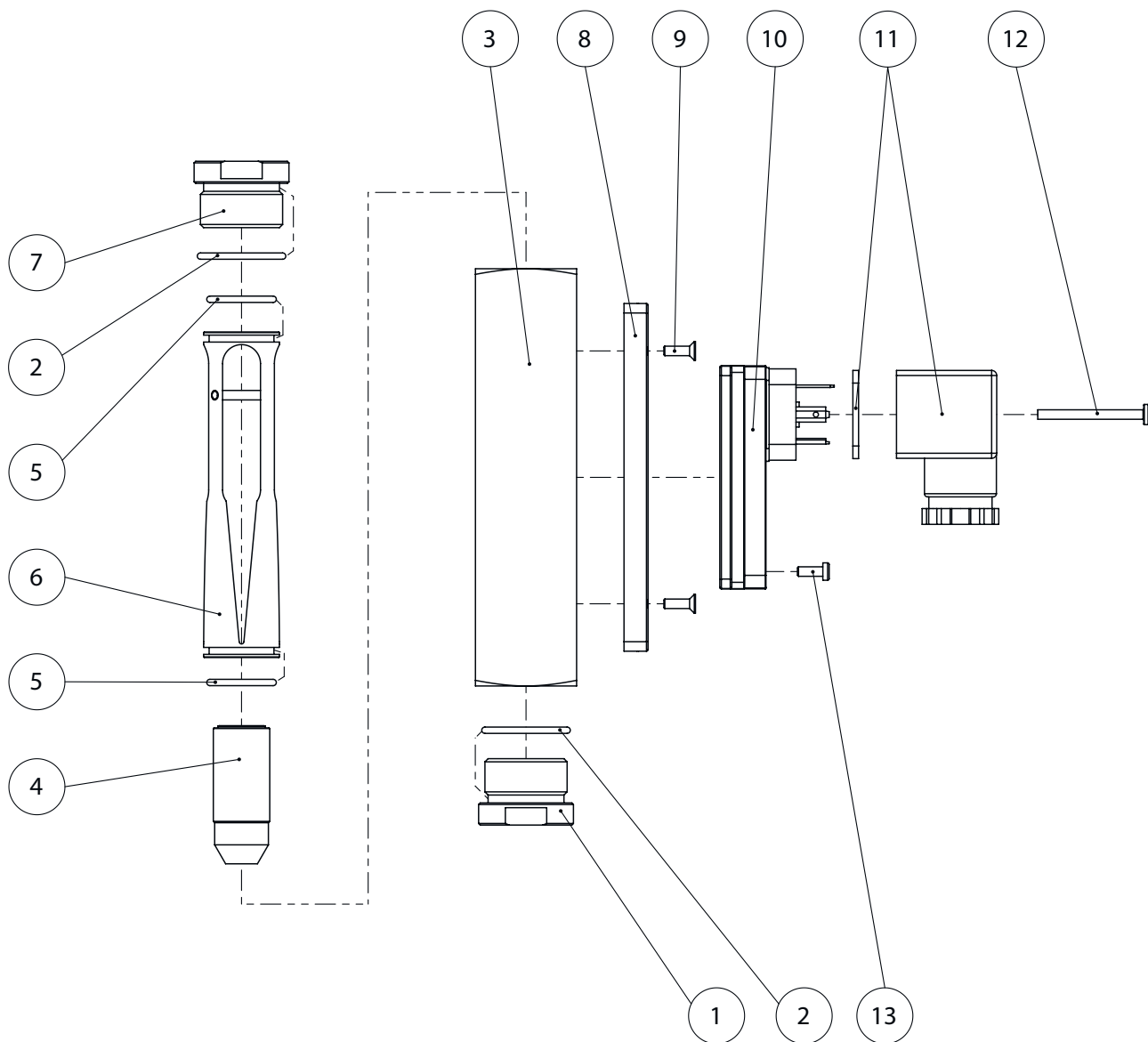
Fig. 70: EZ__DWM-18 SG-30
