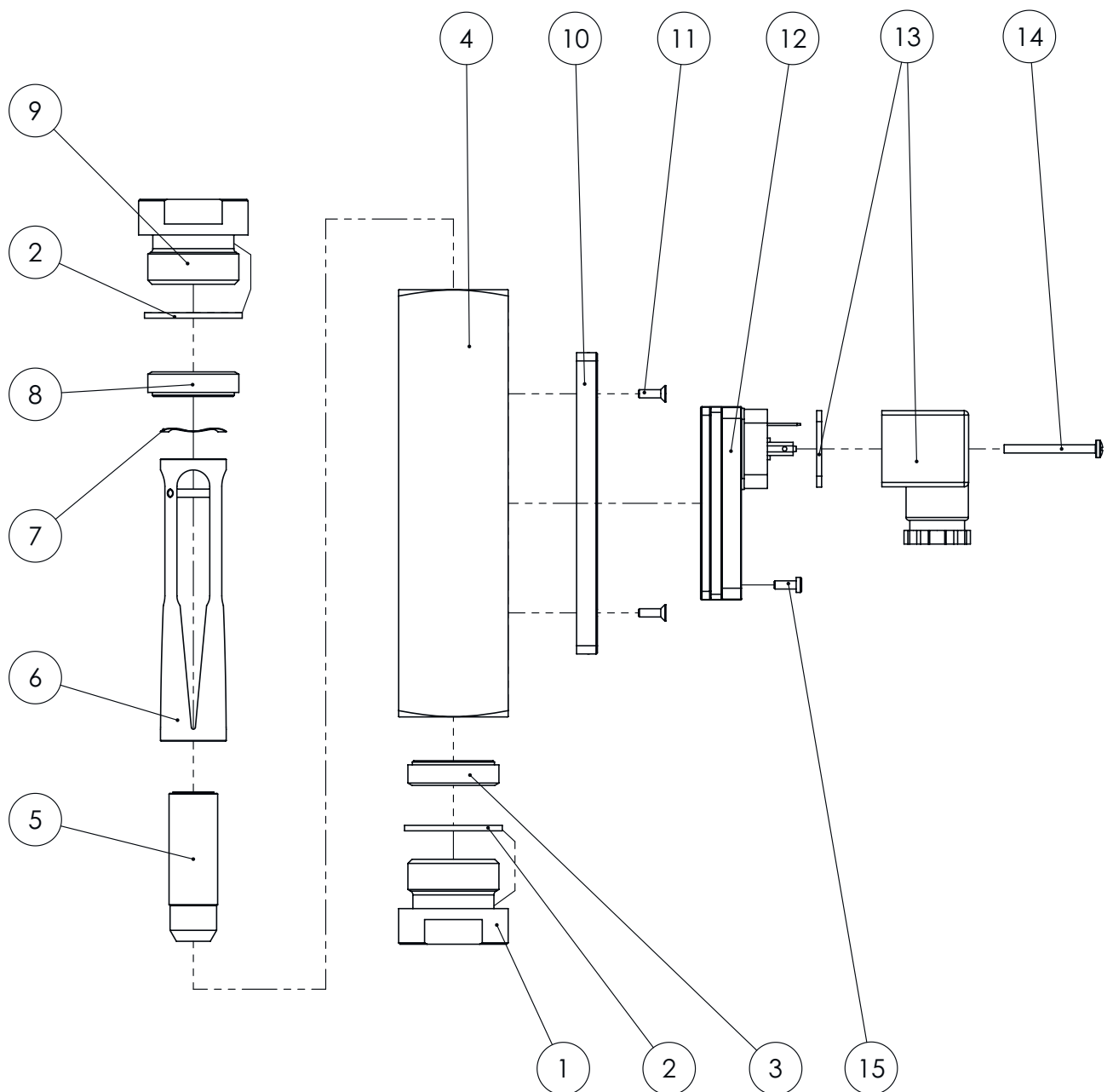
Fig. 71: EZ_DWM-50 SG-30
