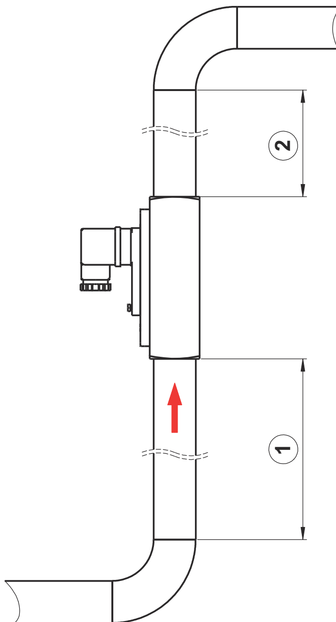
Fig. 8: Strainer
