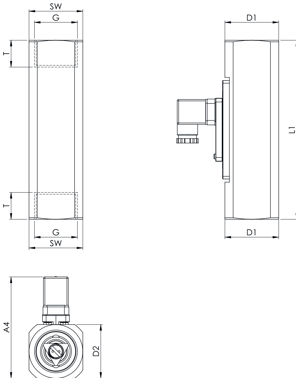
Fig. 70: Typ DUM 150-250
