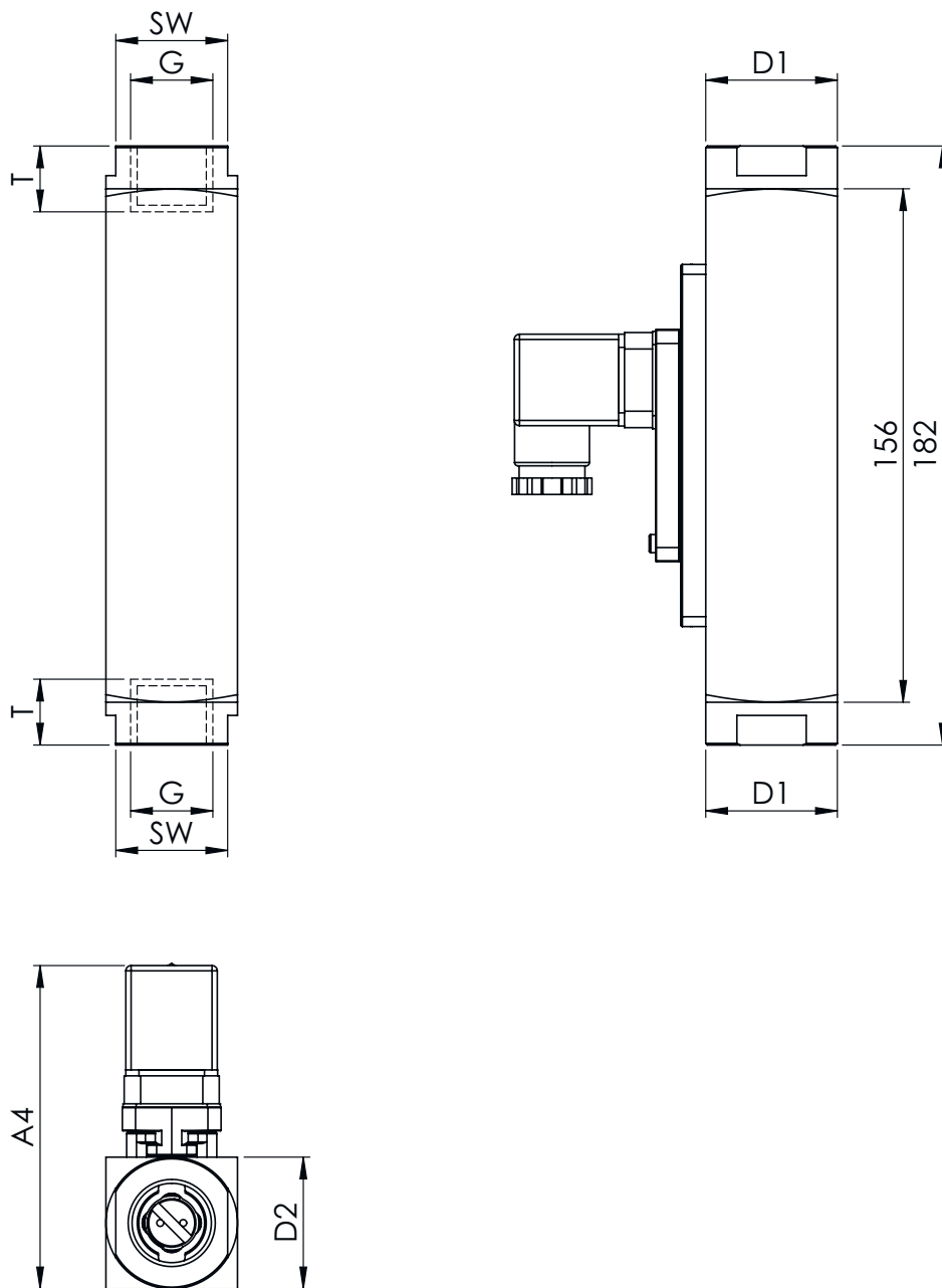
Fig. 69: Typ DUM 70-110
