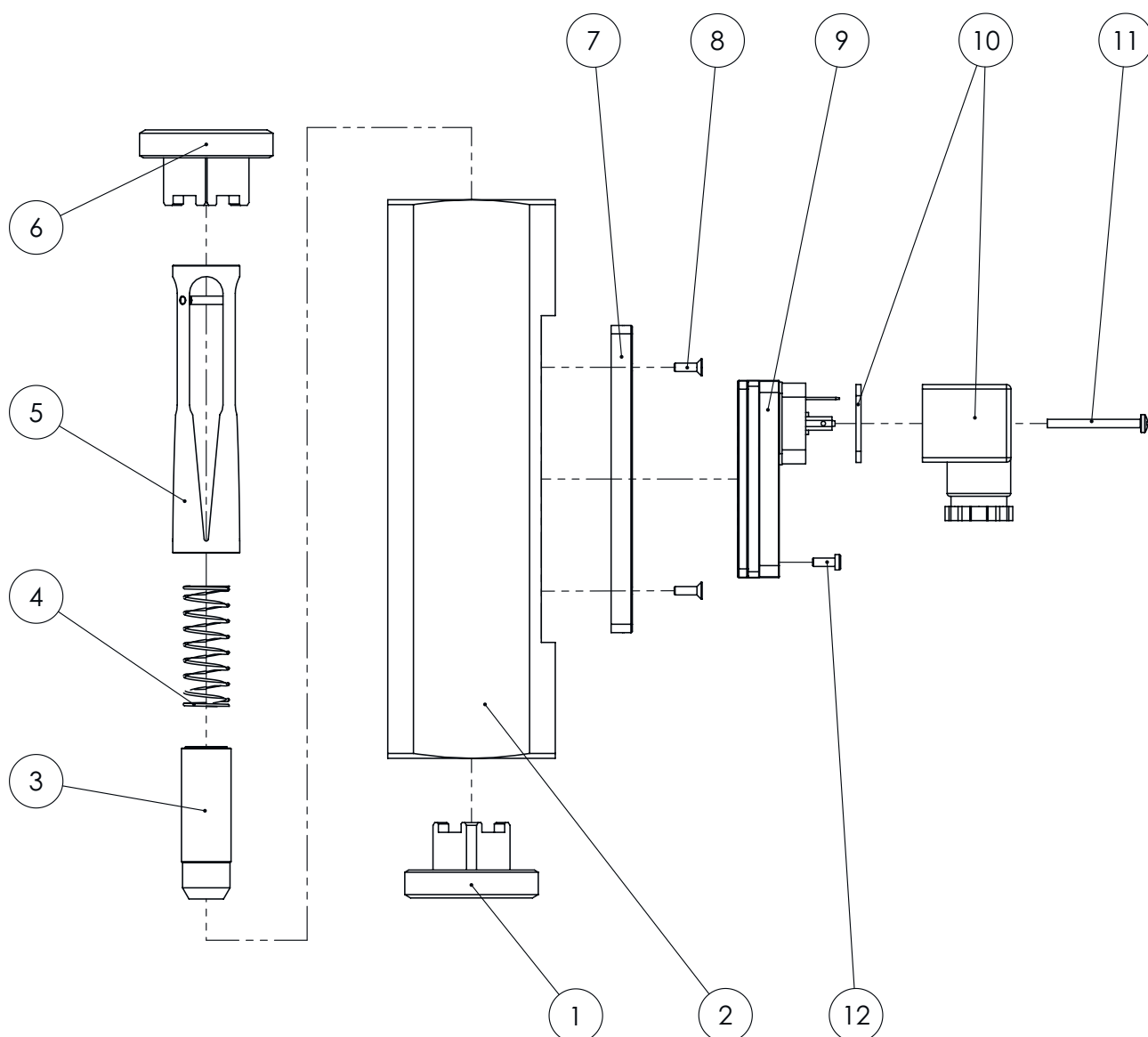
Fig. 73: EZ_DUM 150-250 G1 1_2 SG-30
