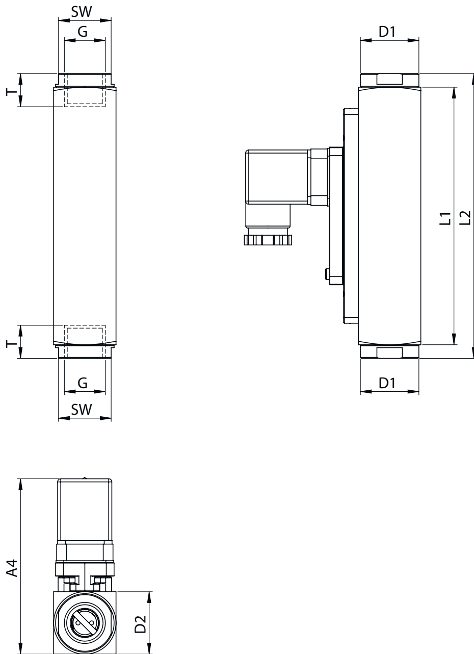
Fig. 68: Typ DUM 4-55
