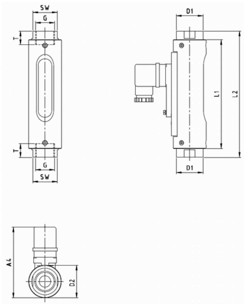
Fig. 75: Dimension sheet
