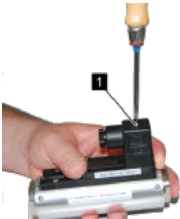
Fig. 27: Detach socket
