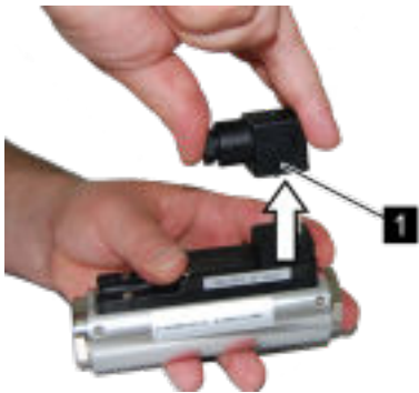
Fig. 28: Remove socket
