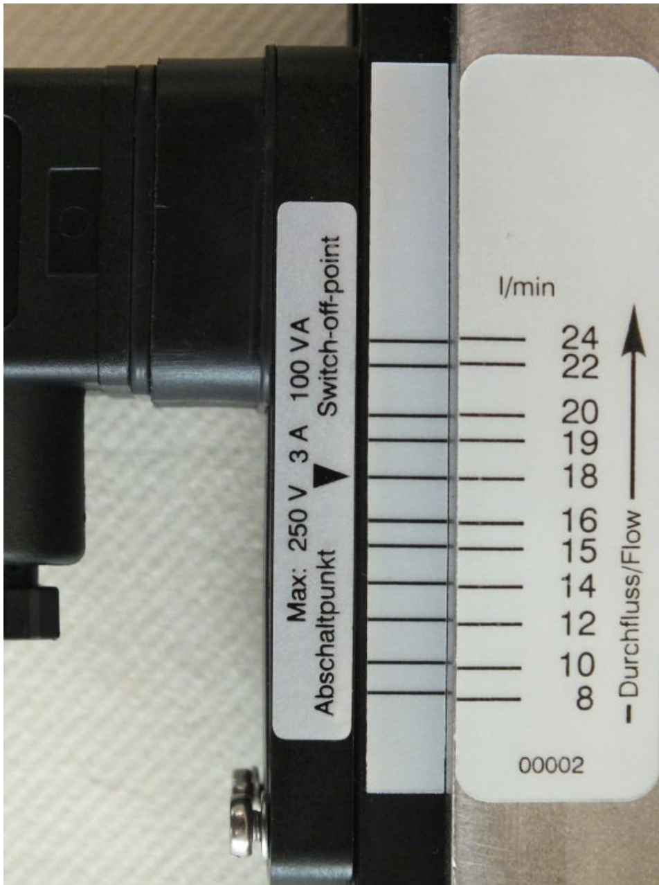
Abb. 4: Körperskala DKME/A-1
