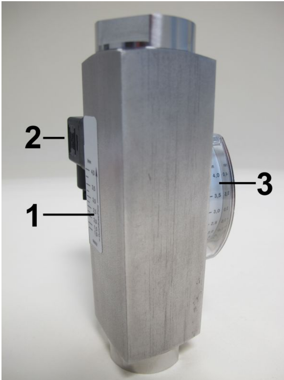
Abb. 1: Strömungswächter DKME/A-1
