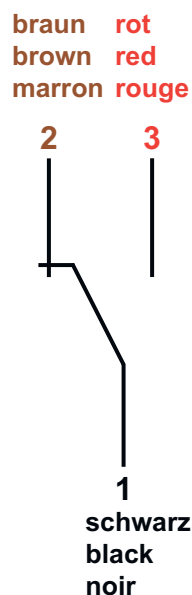
Abb. 26: Zustand des Kontaktes bei Gerät ohne Durchfluss
