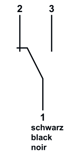
Abb. 24: Zustand des Kontaktes bei Gerät ohne Durchfluss
