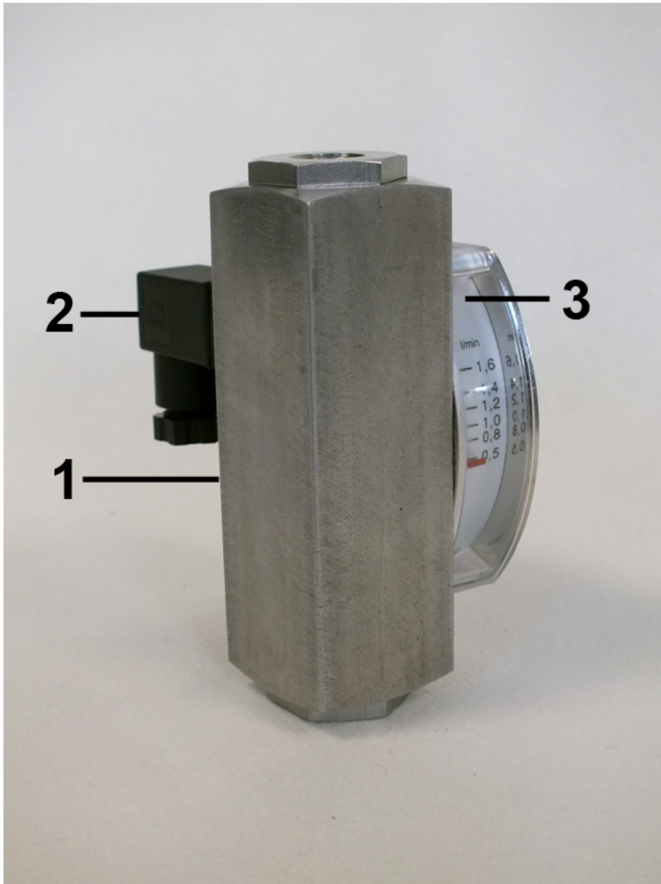
Abb. 1: Strömungswächter DKM/A-2
