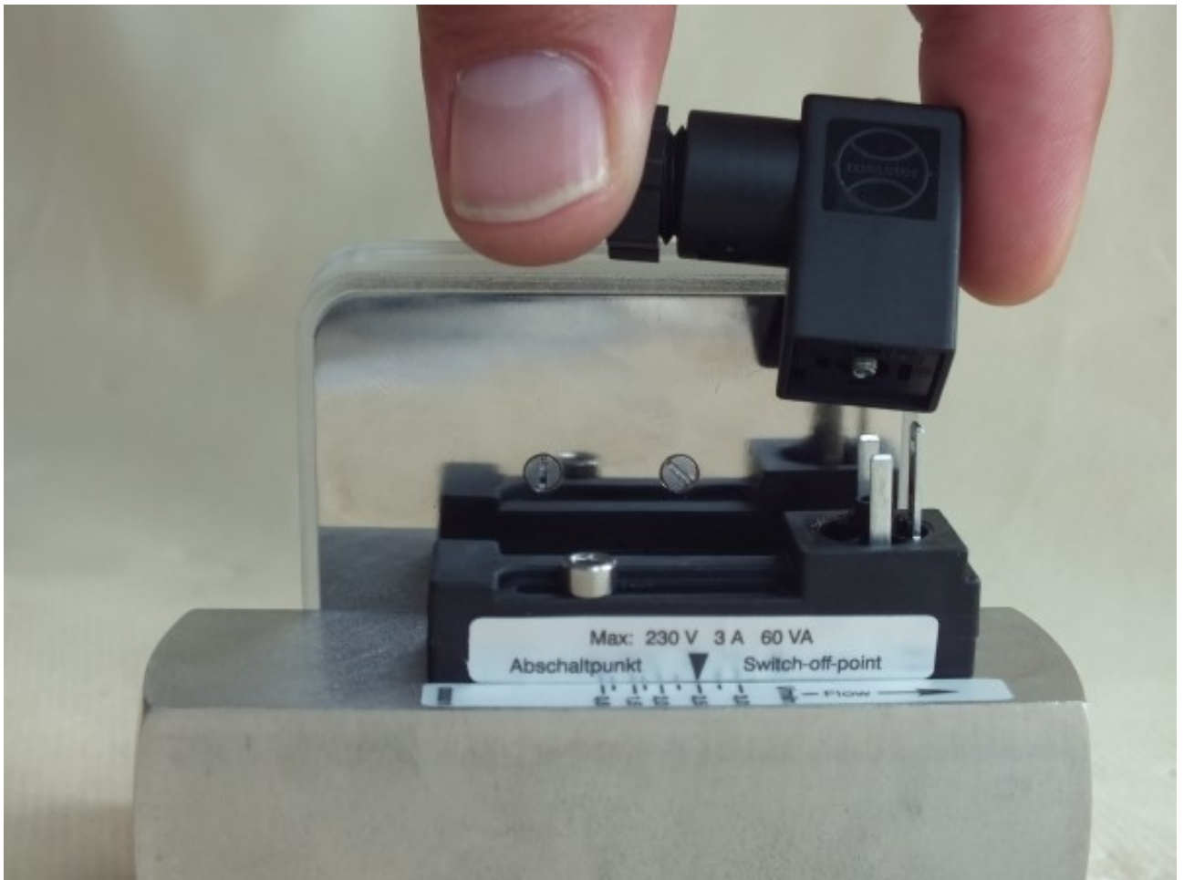
Abb. 68: Steckerdose abziehen
