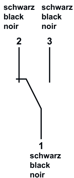
Abb. 24: Zustand des Kontaktes bei Gerät ohne Durchfluss
