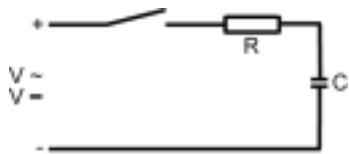
Abb. 34: Schutzmaßnahme bei kapazitiver Belastung
