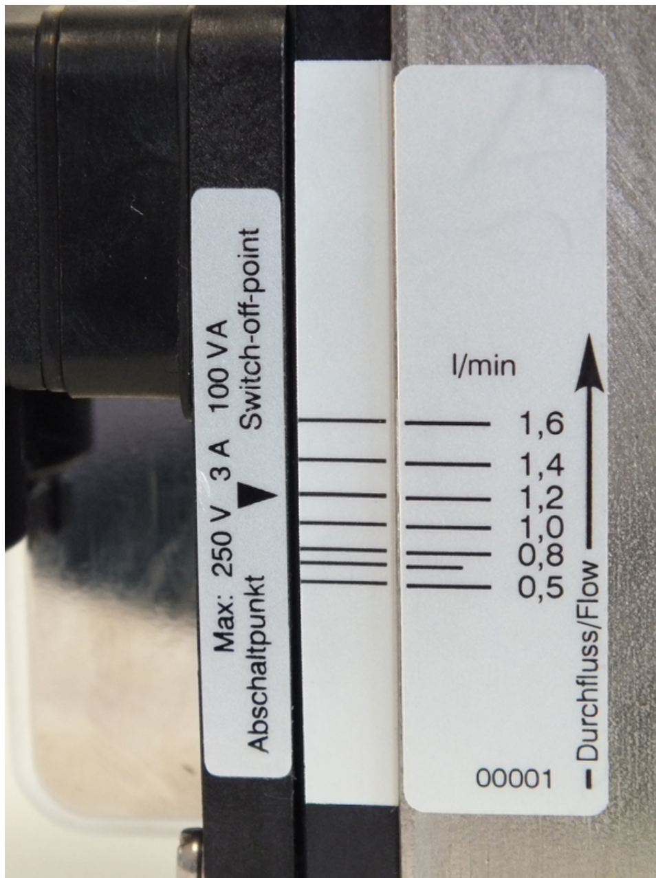
Abb. 4: Körperskala DKM/A-2 30x70
