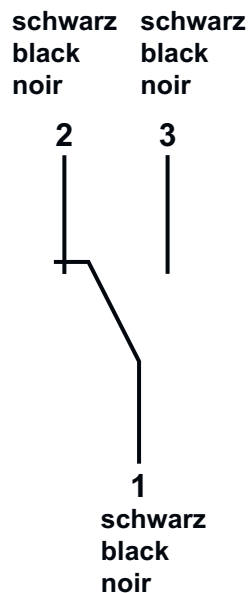
Abb. 23: Zustand des Kontaktes bei Gerät ohne Durchfluss
