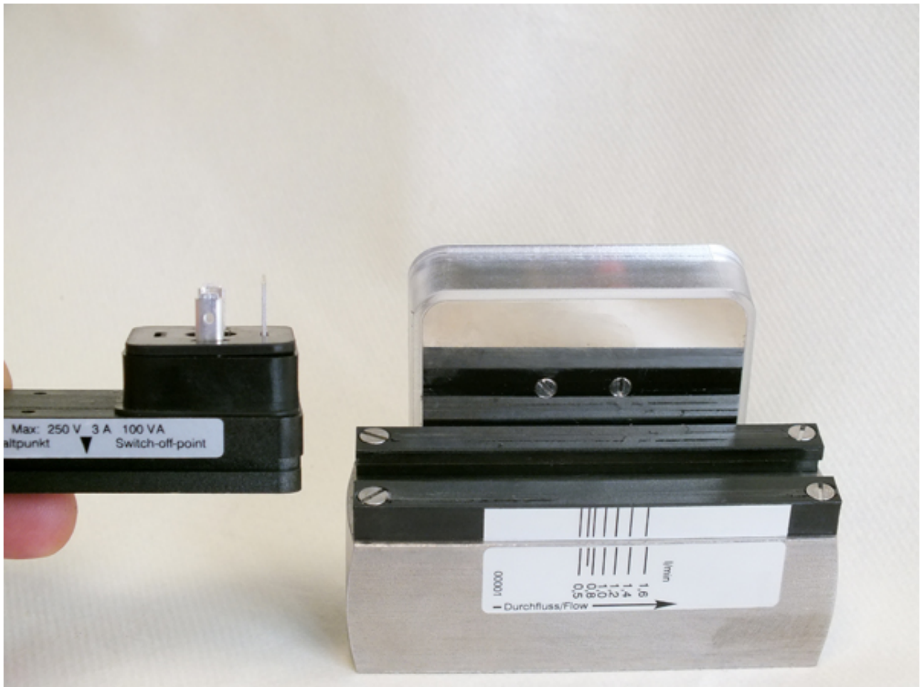
Abb. 75: Schaltkontakt abnehmen
