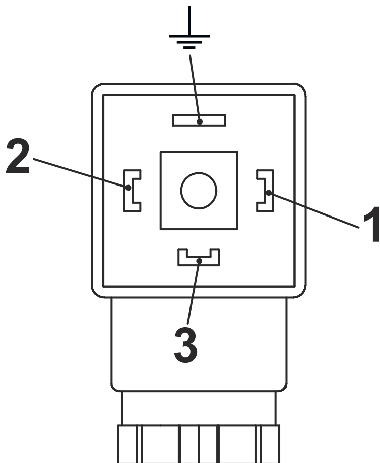
Abb. 17: Pin-Belegung Steckerdose Wechsler (Erde-Anschluss nicht genutzt)
