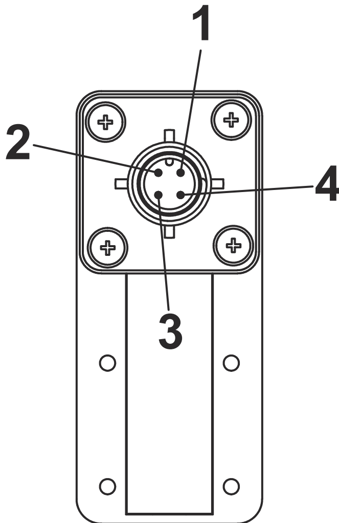
Abb. 18: Pin-Belegung Gerätestecker M12x1
