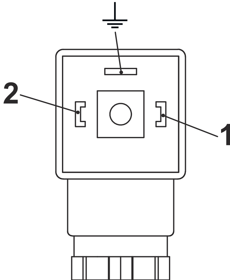
Abb. 15: Pin-Belegung Steckerdose Schließer (Erde-Anschluss nicht genutzt)
