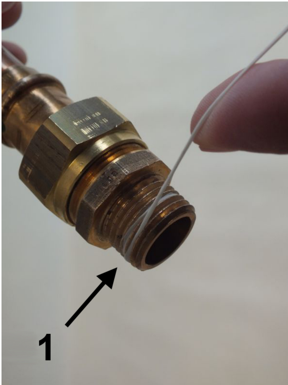
Abb. 9: Dichtfaden aufbringen
