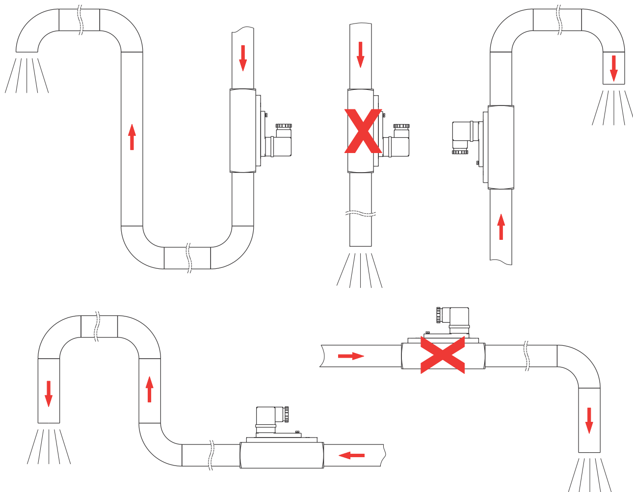
Abb. 7: Freier Auslauf
