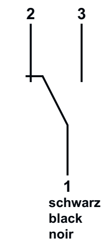
Abb. 23: Zustand des Kontaktes bei Gerät ohne Durchfluss
