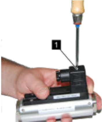
Abb. 64: Steckerdose lösen
