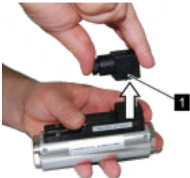
Abb. 65: Steckerdose abziehen
