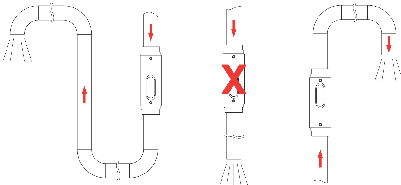
Abb. 7: Freier Auslauf
