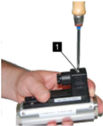
Abb. 27: Steckerdose lösen
