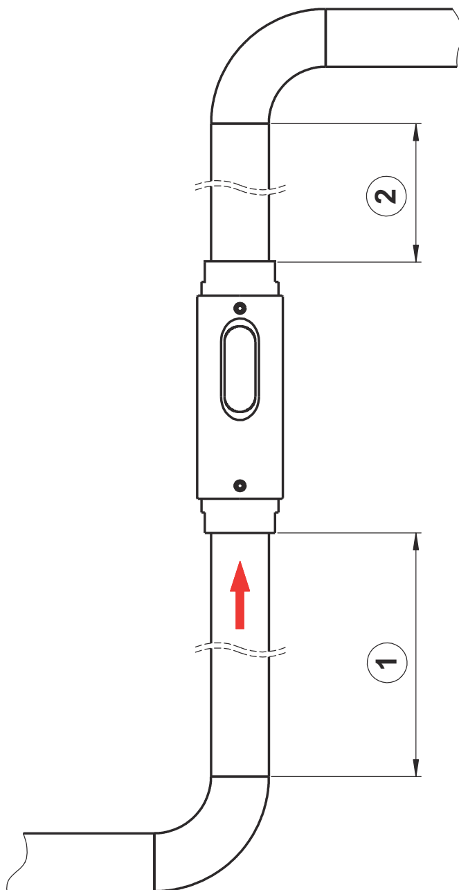
Abb. 6: Beruhigungsstrecken
