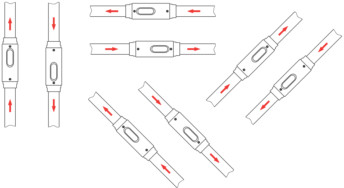
Abb. 5: Einbauposition/Durchflussrichtung
