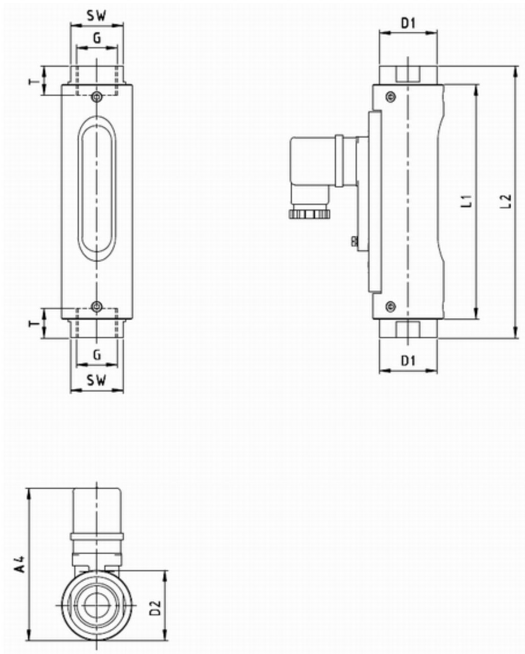
Abb. 75: Maßblatt
