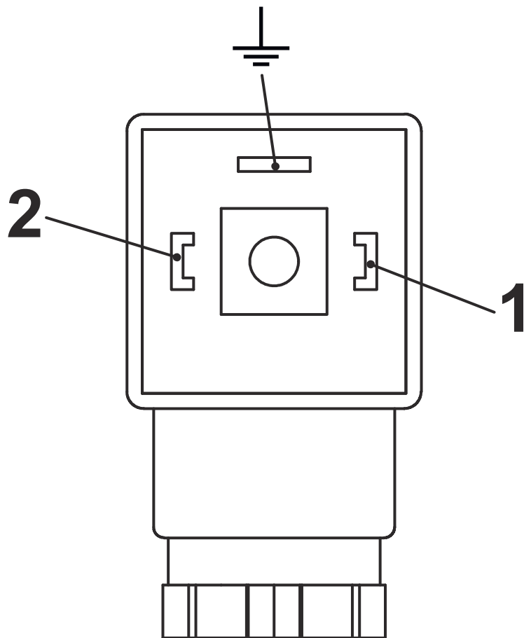
Abb. 14: Pin-Belegung Steckerdose Schließer (Erde-Anschluss nicht genutzt)
