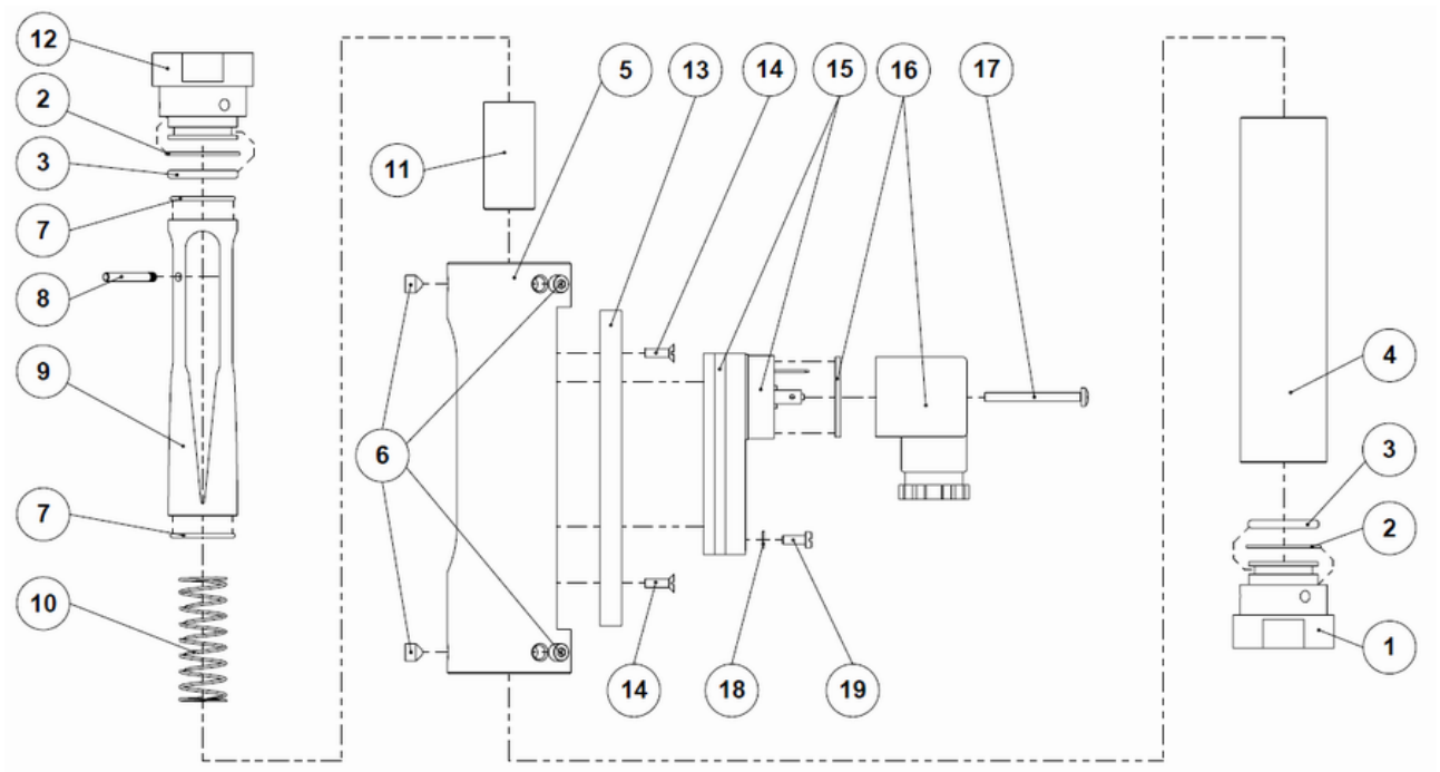
Abb. 76: Ersatzteilzeichnung
