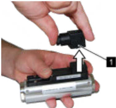
Abb. 28: Steckerdose abziehen
