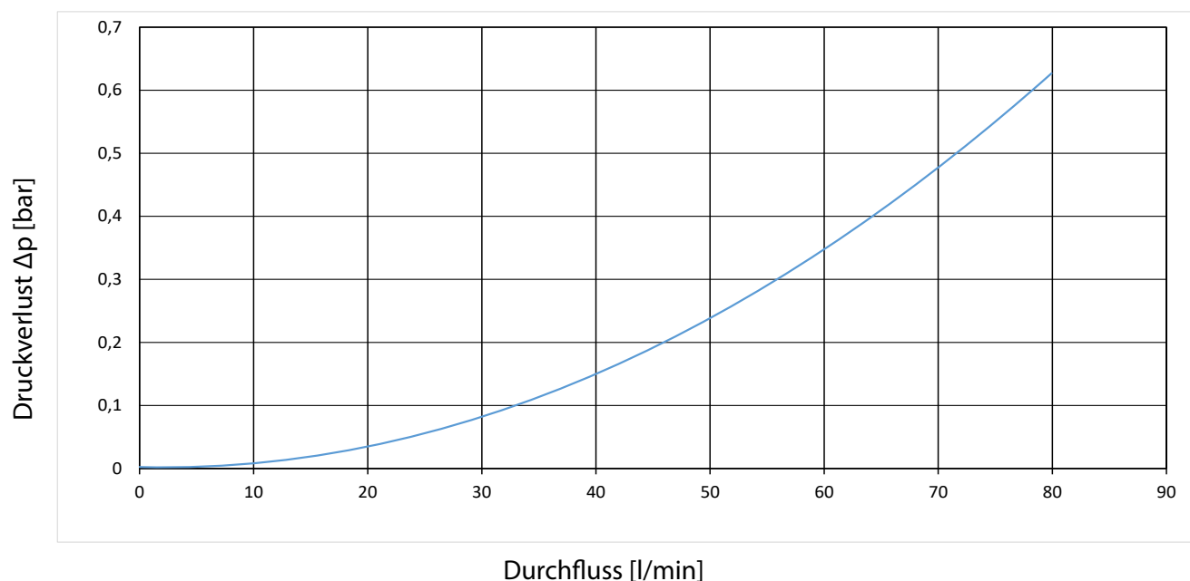
Druckverlustdiagramm
