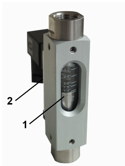
Abb. 1: Strömungswächter RVO/U-4
