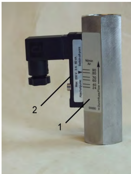
Abb. 1: Strömungswächter RVM/U-L2
