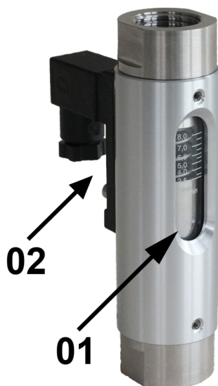
Abb. 1: Strömungswächter DKG-2
