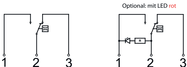
Abb. 3: Anschlussbilder
