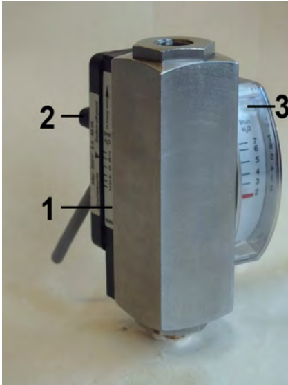
Fig. 1: RVM/UA-2 30x70 flow monitor
