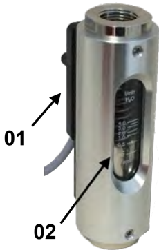
Abb. 1: Strömungswächter DUG
