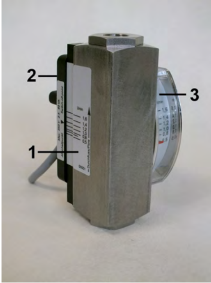
Abb. 1: Strömungswächter DKM/A-2 30x70
