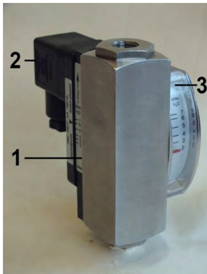
Abb. 1: Strömungswächter RVM/UA-2 30x70
