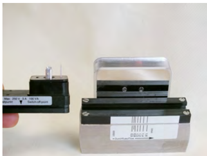
Abb. 72: Schaltkontakt abnehmen
