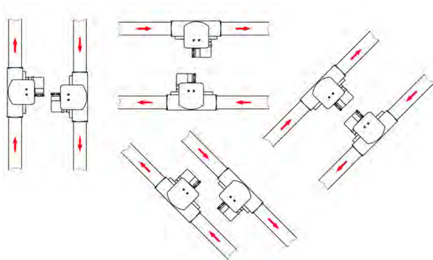
Abb. 6: Einbauposition/Durchflussrichtung
