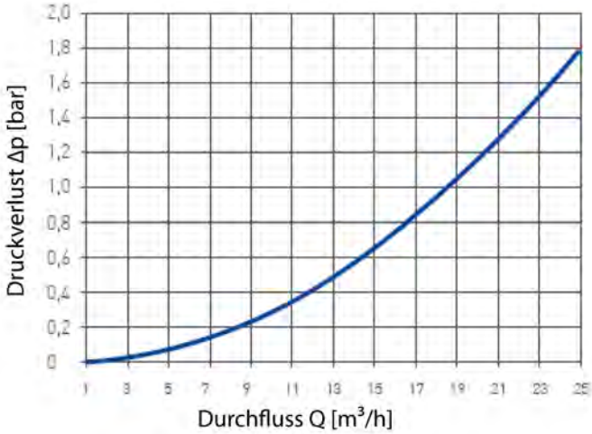
Abb. 7: Druckverlust
