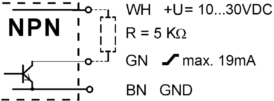
Abb. 3: Anschlussbild
