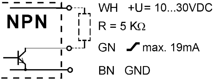
Abb. 8: Anschlussbild
