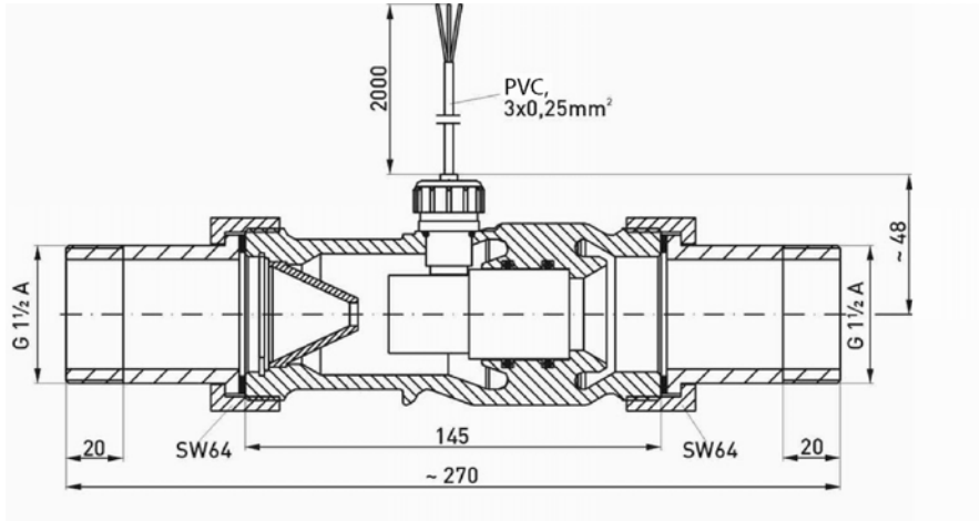
Abb. 6: Maßblatt
