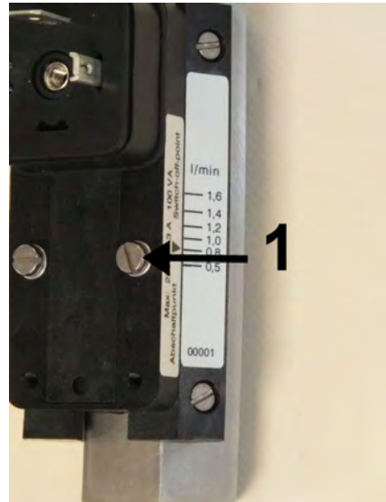
Abb. 31: Feststellschrauben lösen
