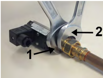
Abb. 11: Gerät einschrauben
