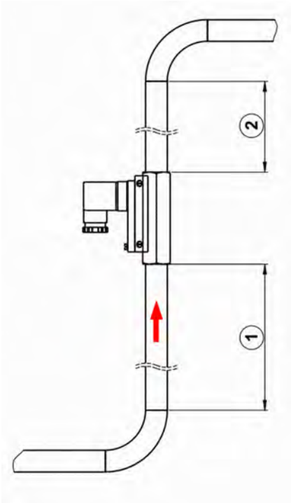
Abb. 6: Beruhigungsstrecken
