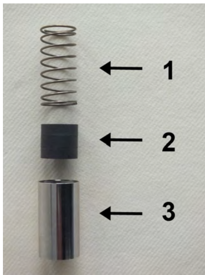
Abb. 47: Innenteile
