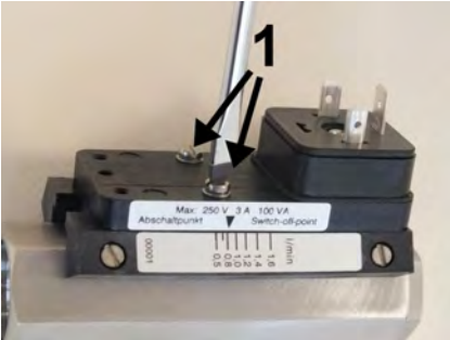
Abb. 56: Feststellschrauben lösen
