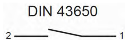
Abb. 13: Zustand des Kontaktes bei Gerät ohne Durchfluss
