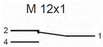
Abb. 19: Zustand des Kontaktes bei Gerät ohne Durchfluss
