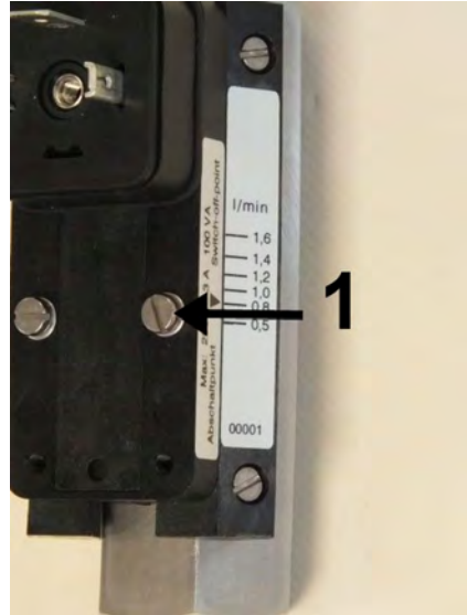
Abb. 32: Feststellschrauben lösen
