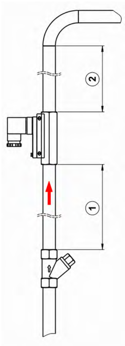
Abb. 8: Schmutzfänger
