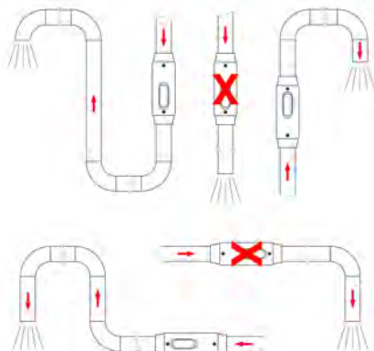
Abb. 7: Freier Auslauf
