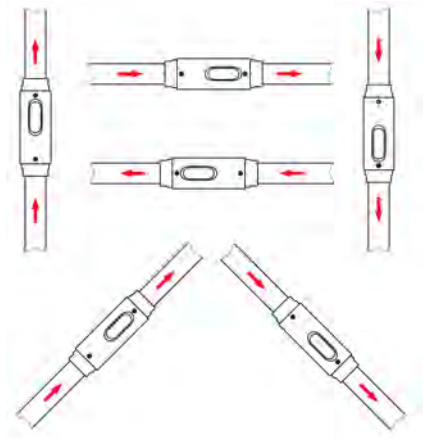
Abb. 5: Einbauposition/Durchflussrichtung
