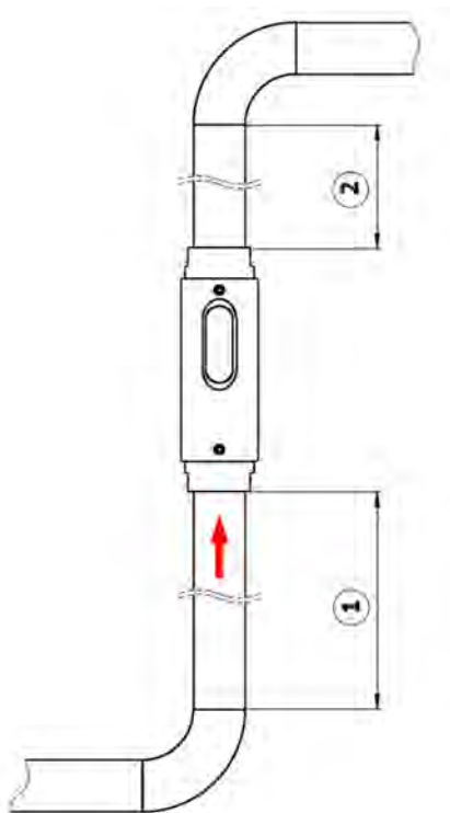
Abb. 6: Beruhigungsstrecken
